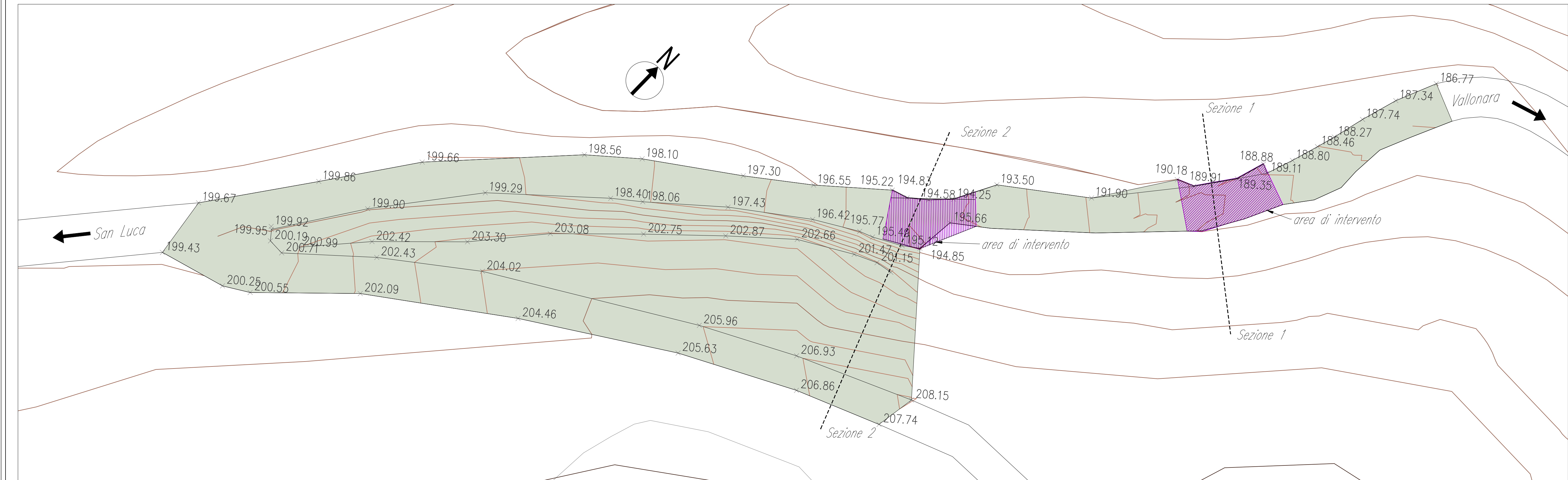
PLANIMETRIA - SCALA 1:200
