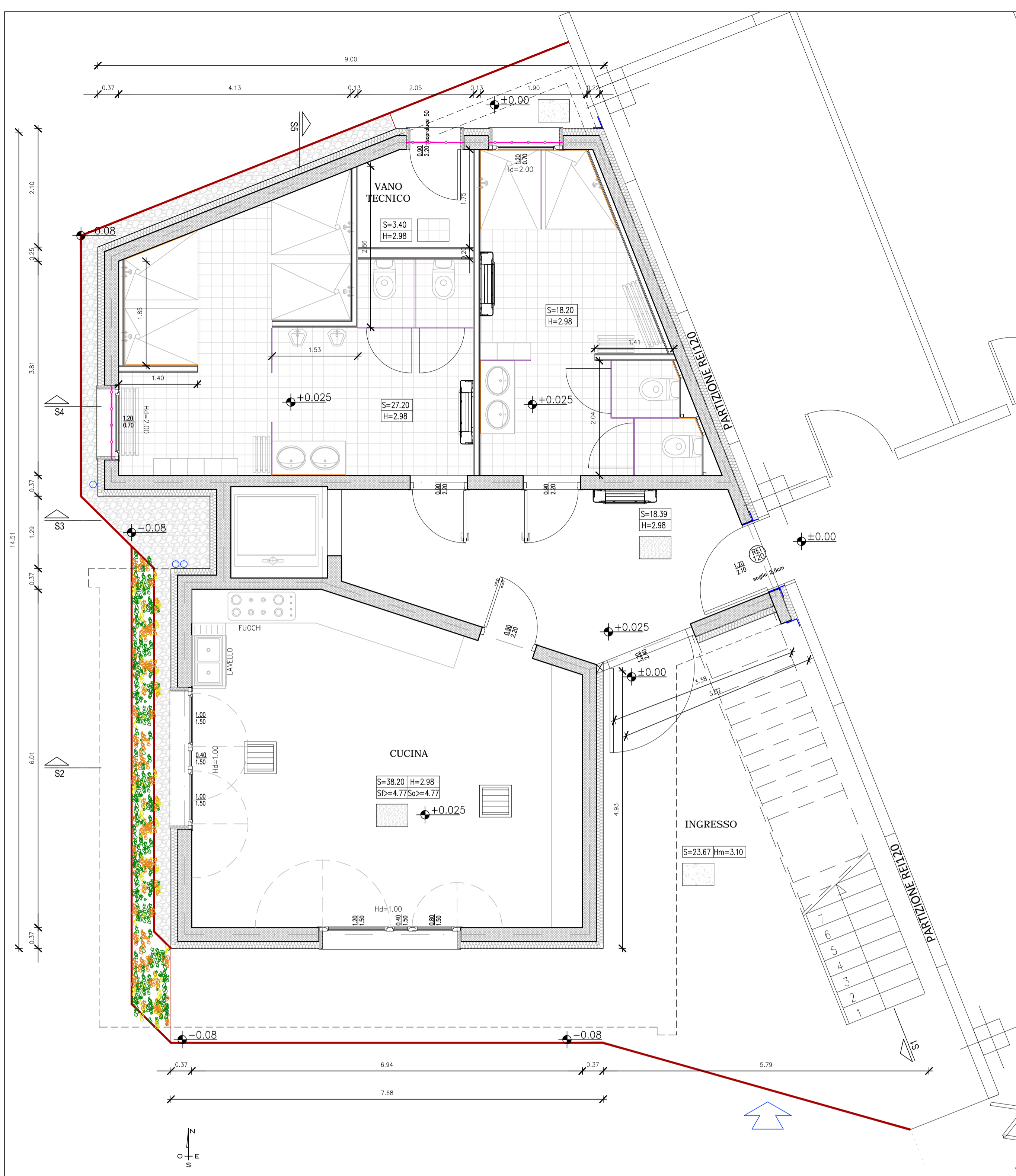
PIANTA PIANO TERRA - 1:50
