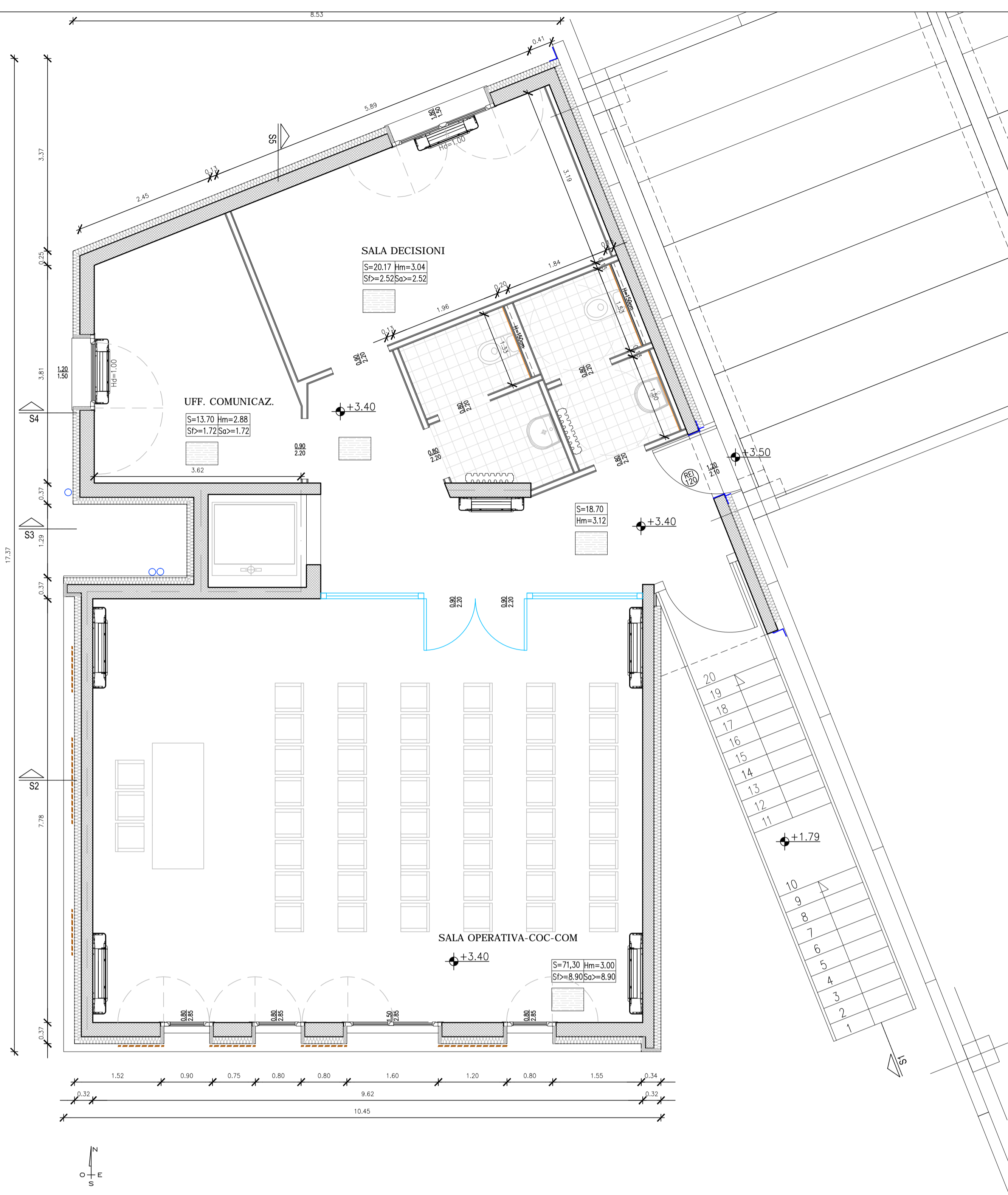
PIANTA PIANO PRIMO - 1:50
