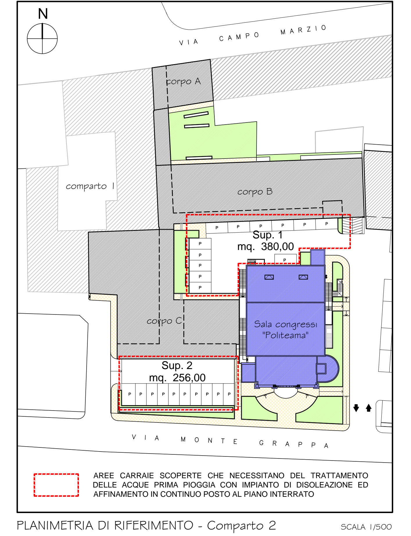
PLANIMETRIA DI RIFERIMENTO - Comparto 2
