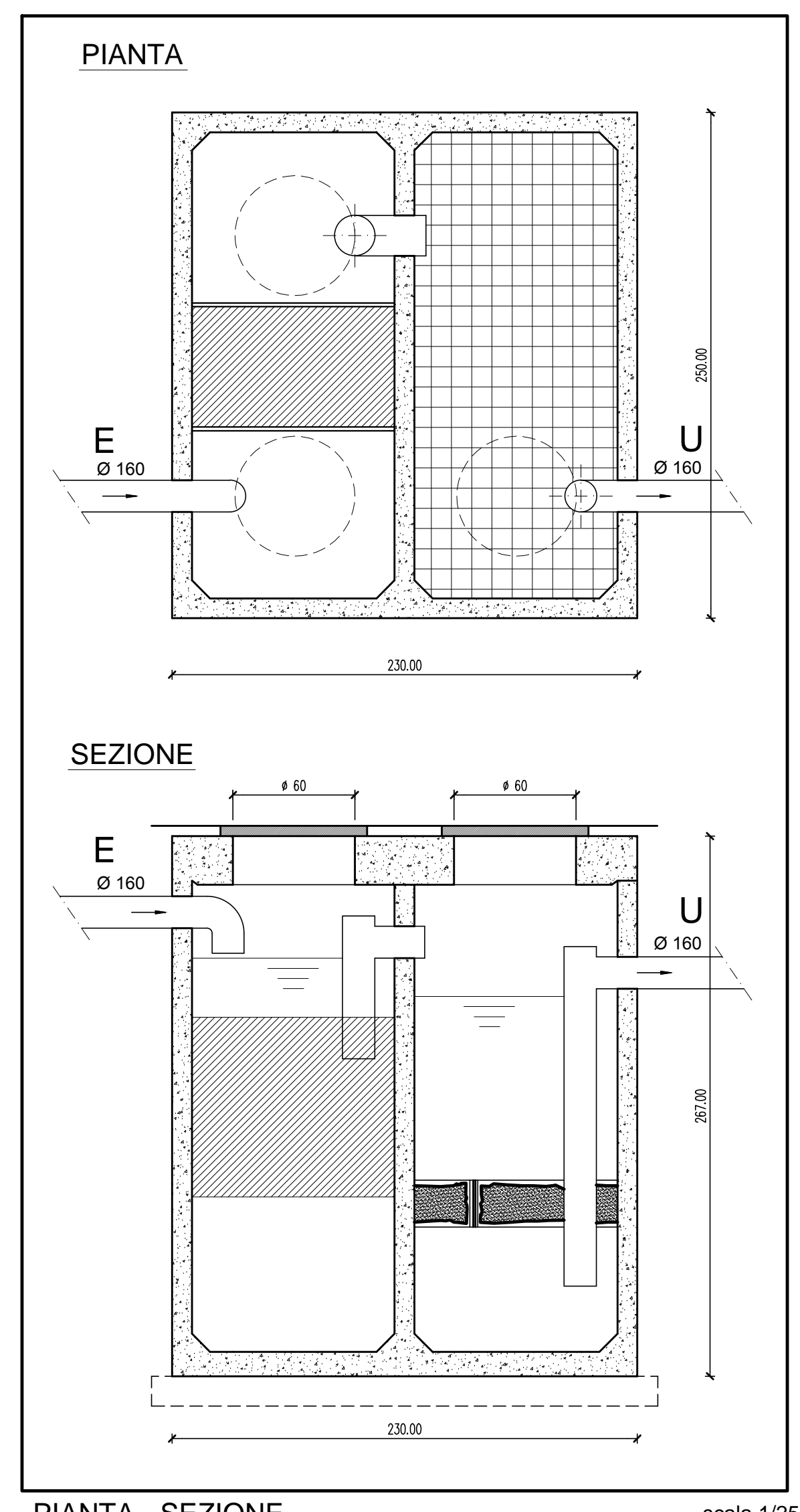
PIANTA - SEZIONE
