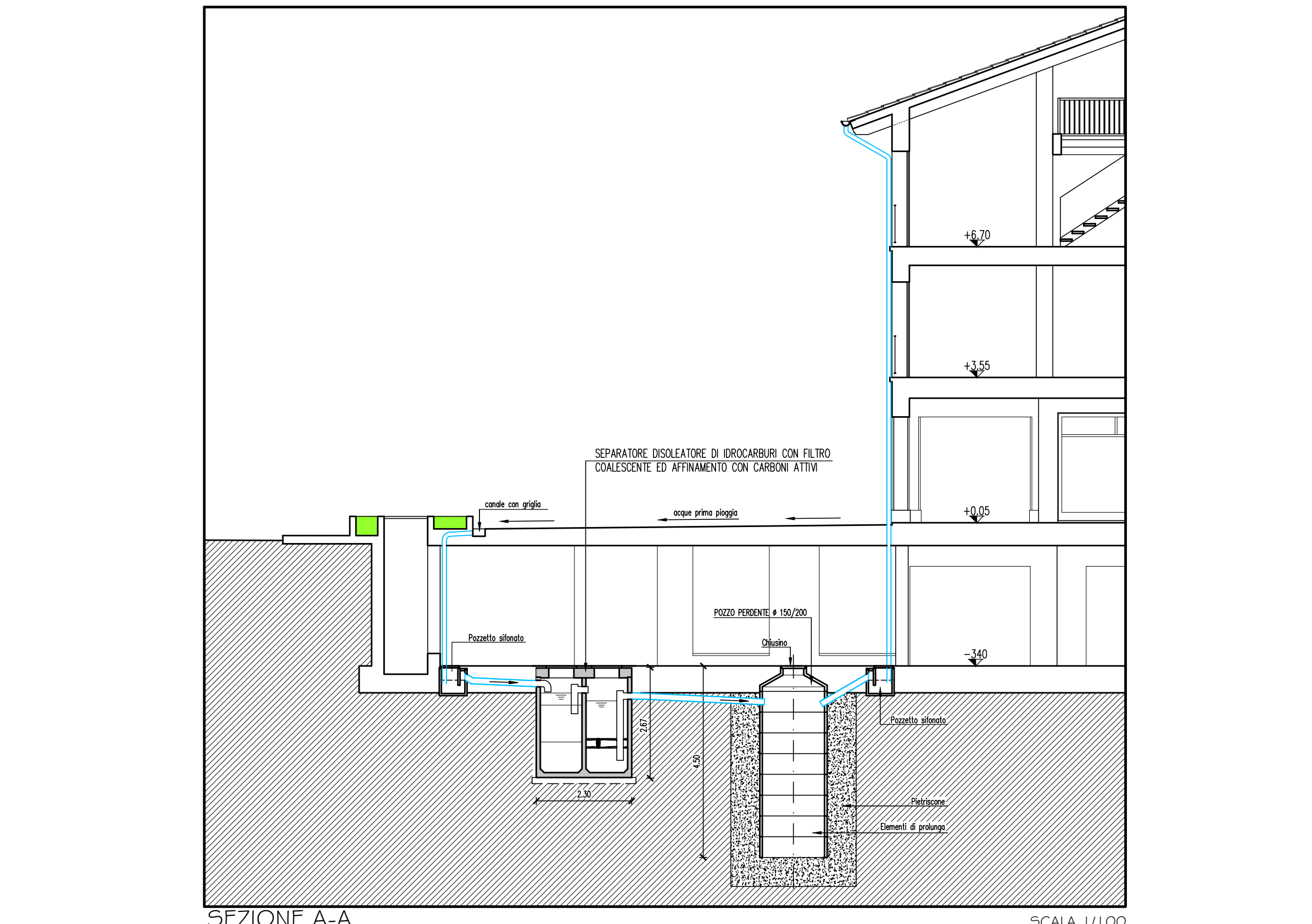
SEZIONE A-A
