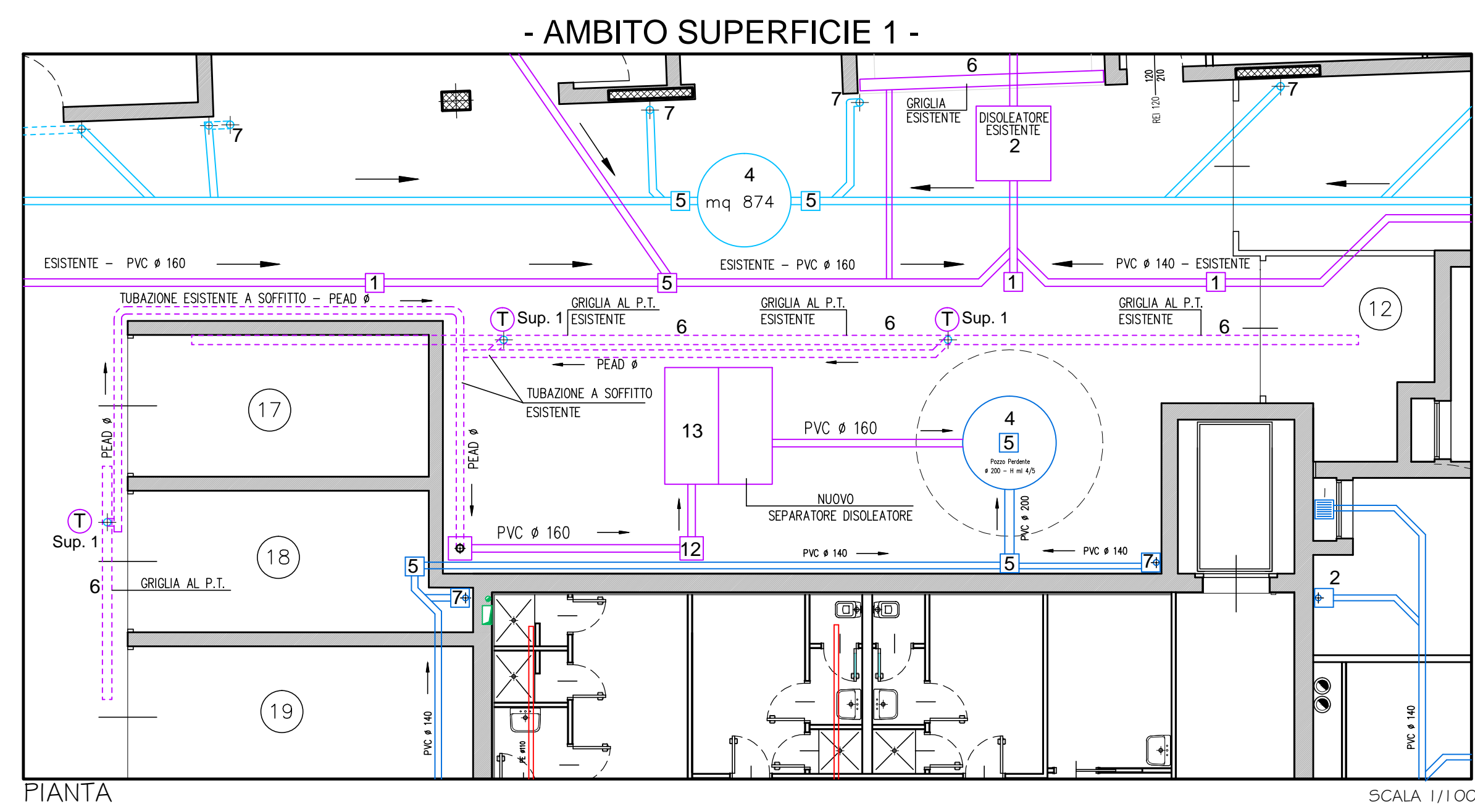
PIANTA - AMBITO SUPERFICIE 1
