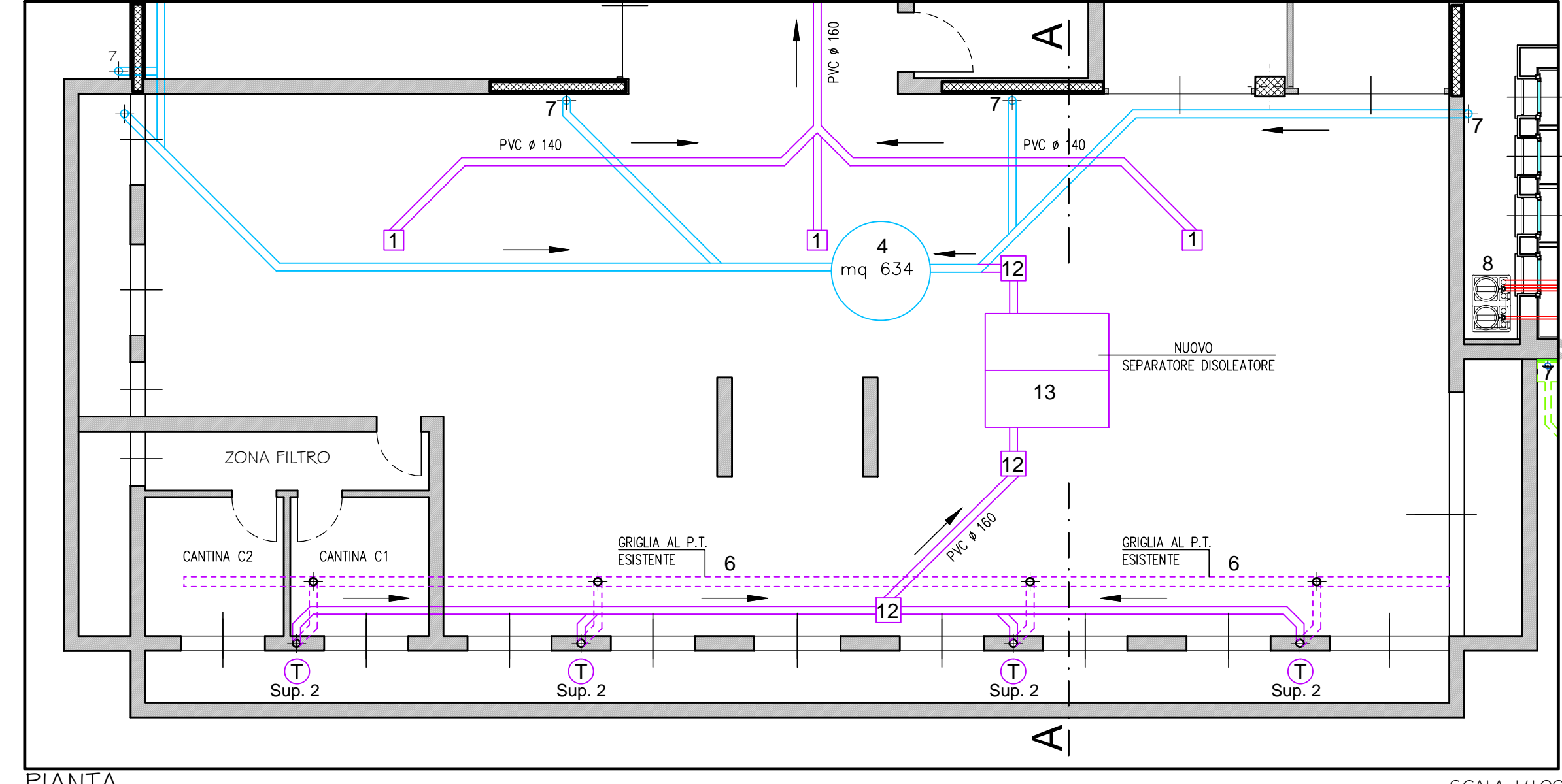
PIANTA - AMBITO SUPERFICIE 2
