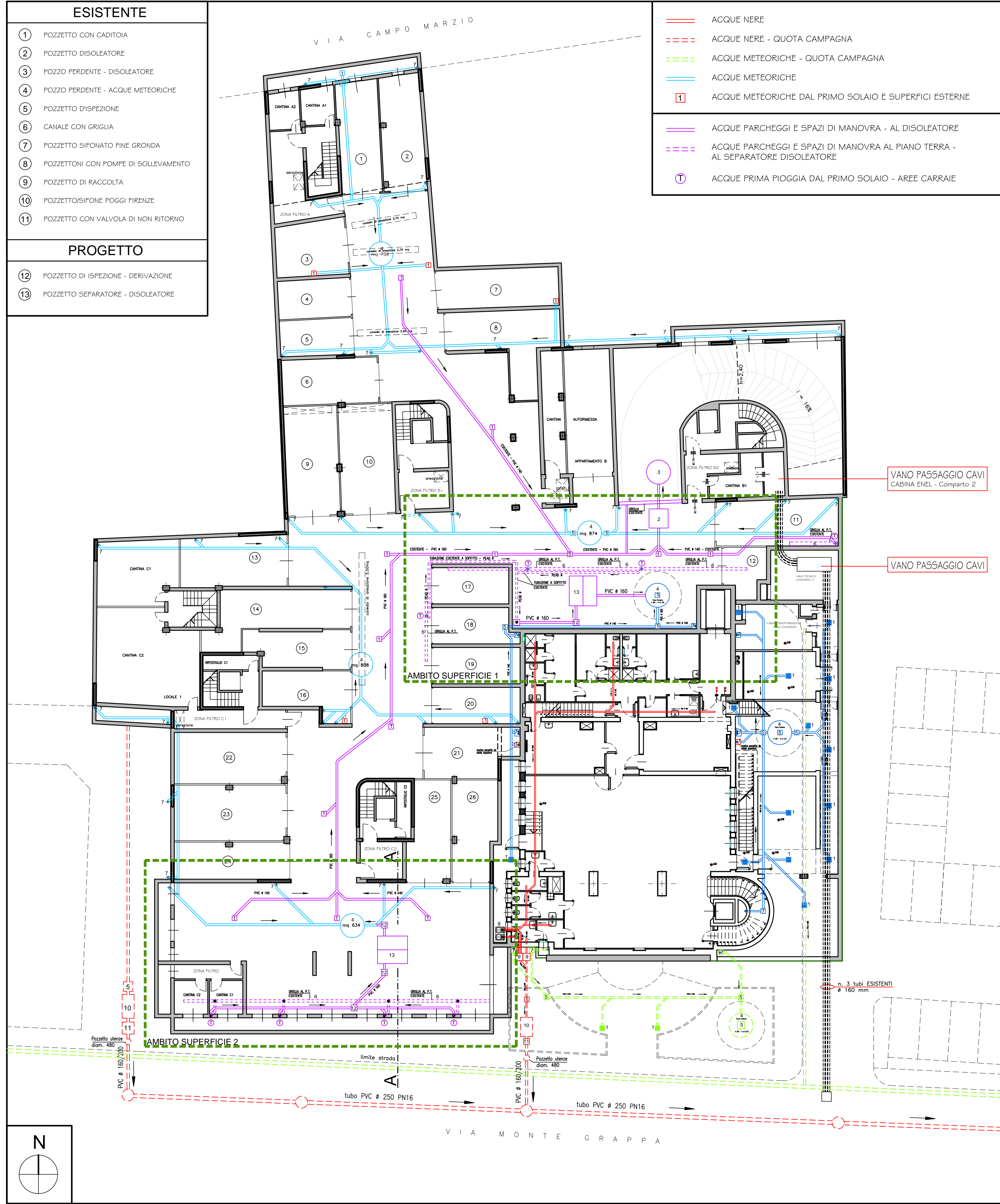
PIANTA PIANO INTERRATO
